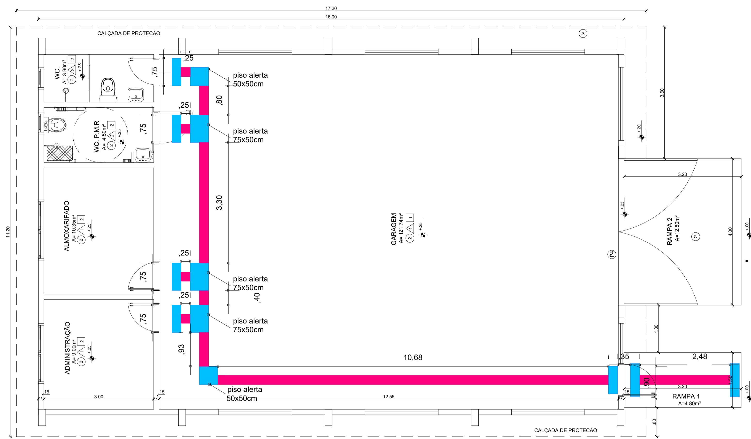
PLANTA BAIXA PROJETO ACESSIBILIDADE ESC 1/50
